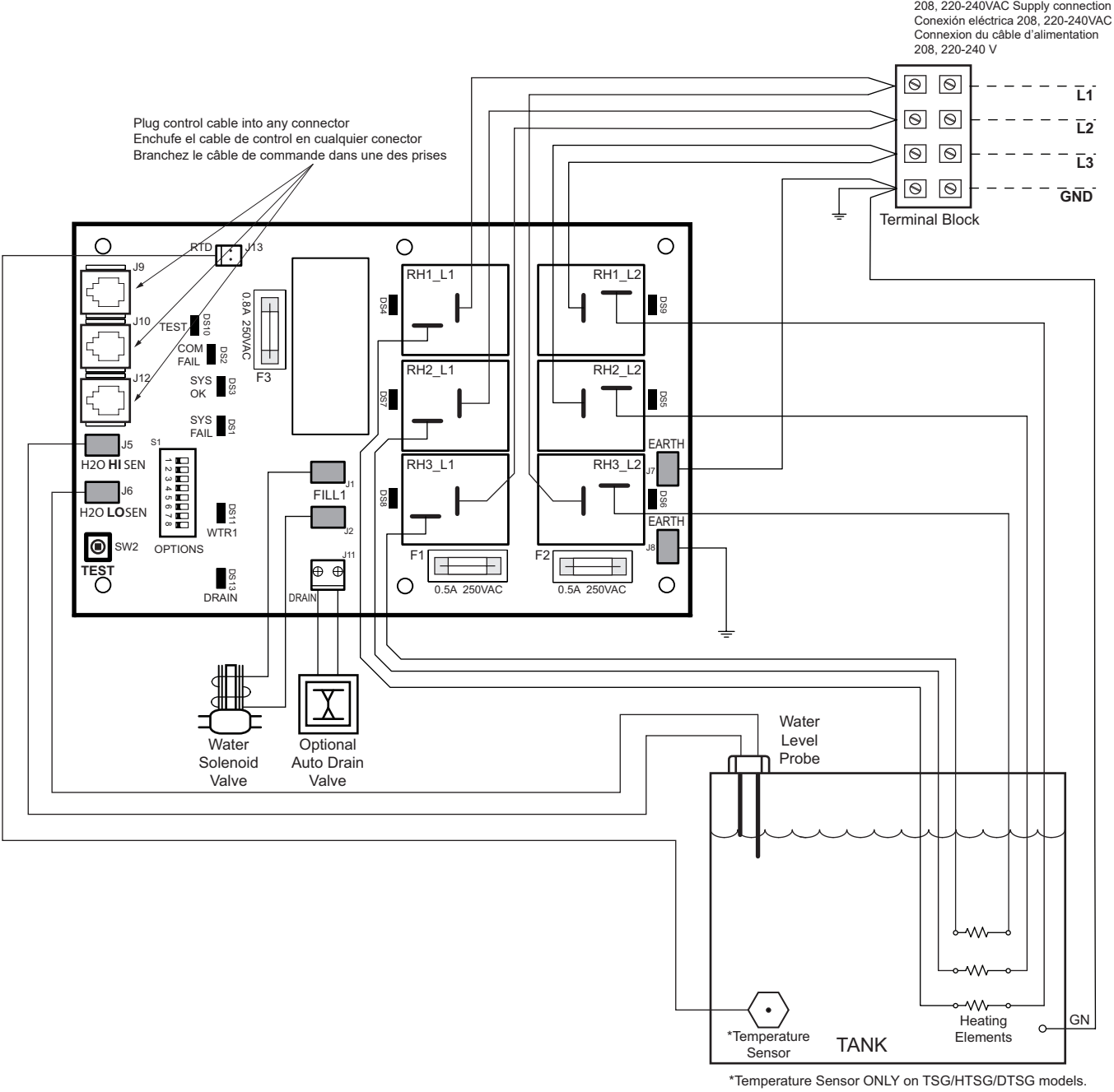
Figure 5 - Schéma de câblage - Trois phases
