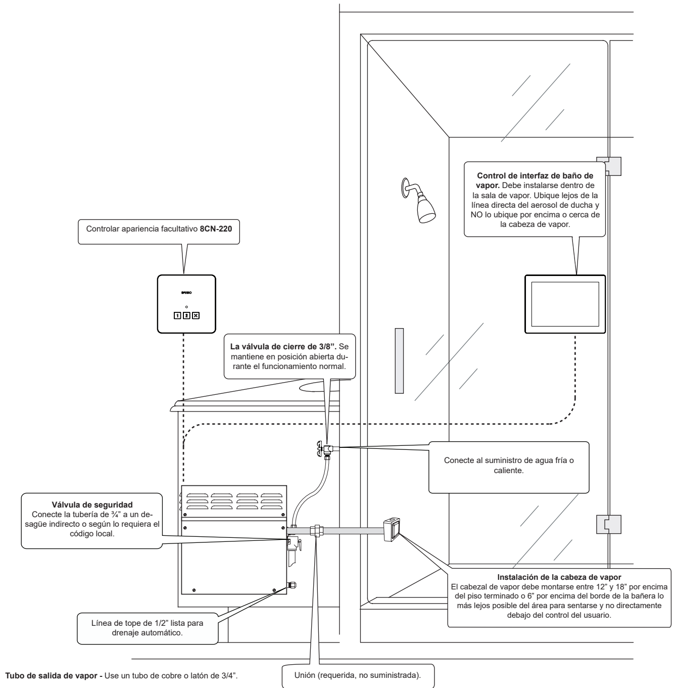
Figure 3 - Instalación típica
